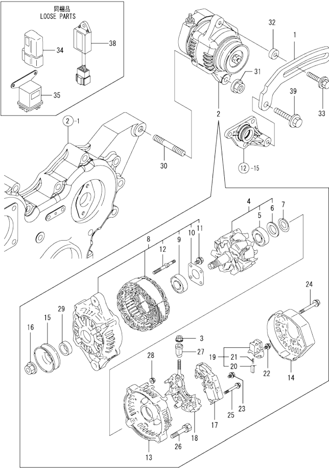
Fig.18. GENERATOR
